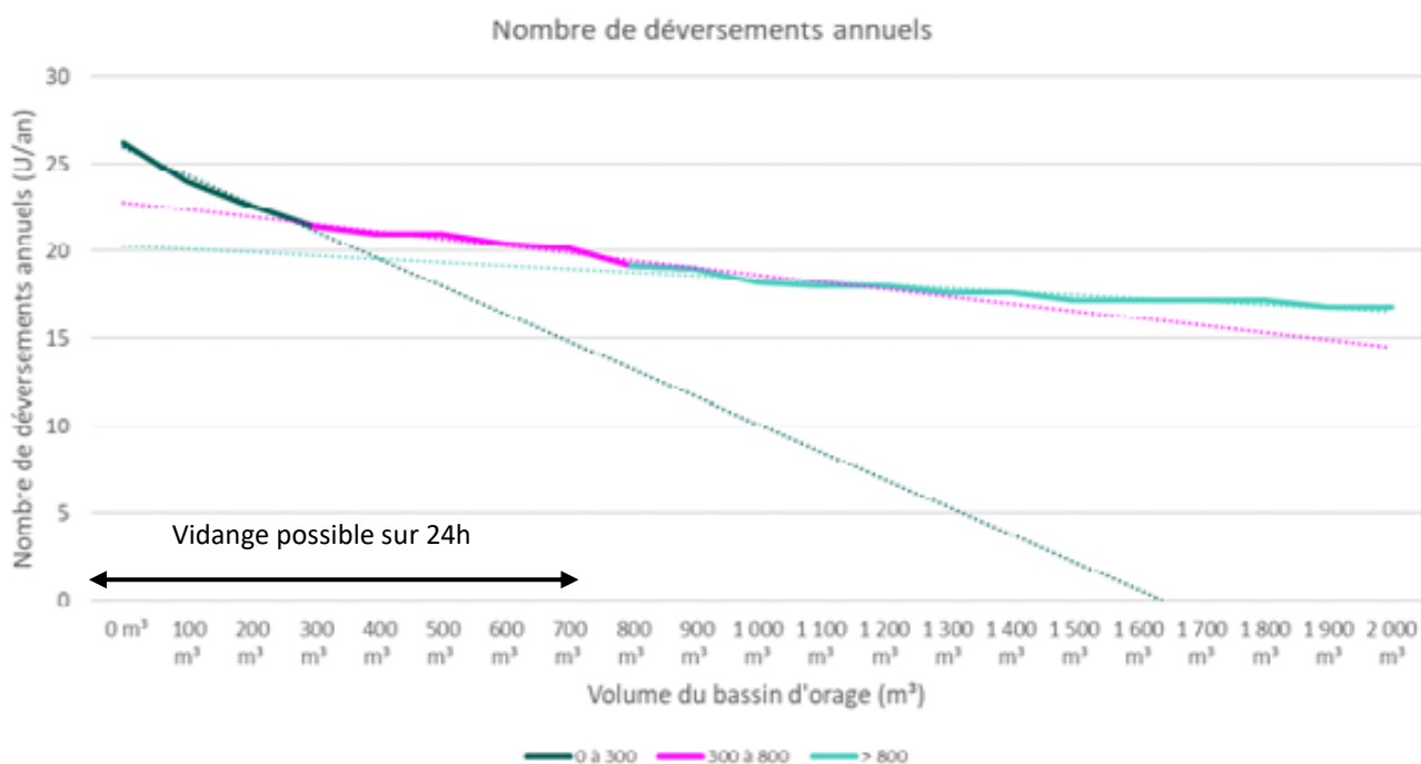
Figure 27 : Influence du bassin d'orage sur le nombre de déversements annuels- Situation actuelle
